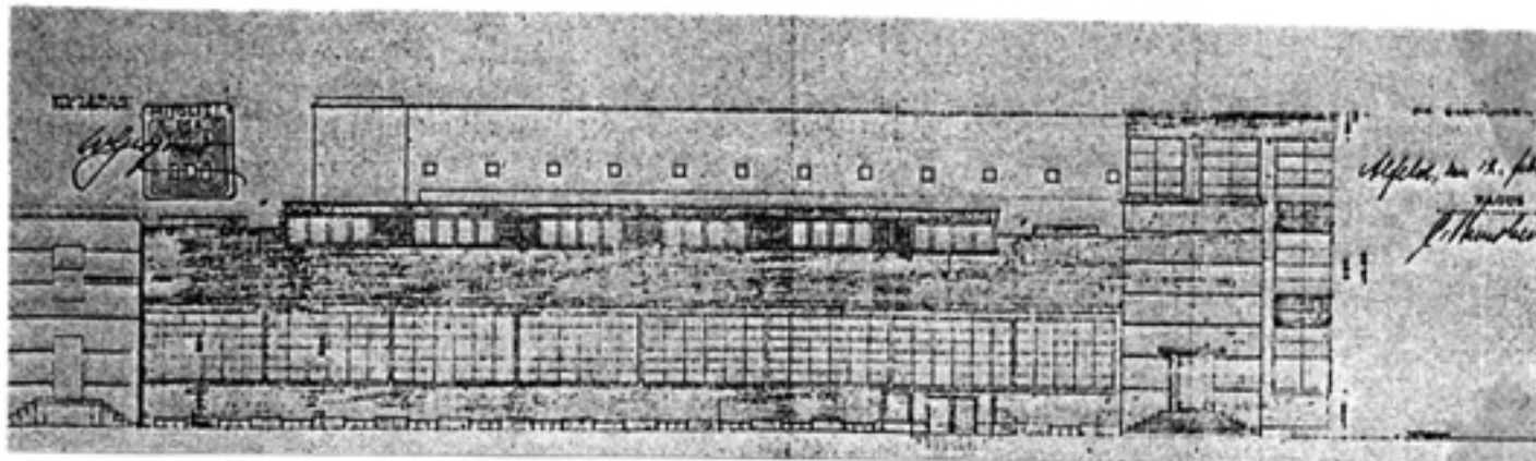
9. ALZADO FRONTAL 1914
