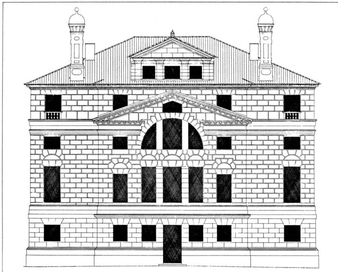
FACHADA HACIA EL JARDIN
