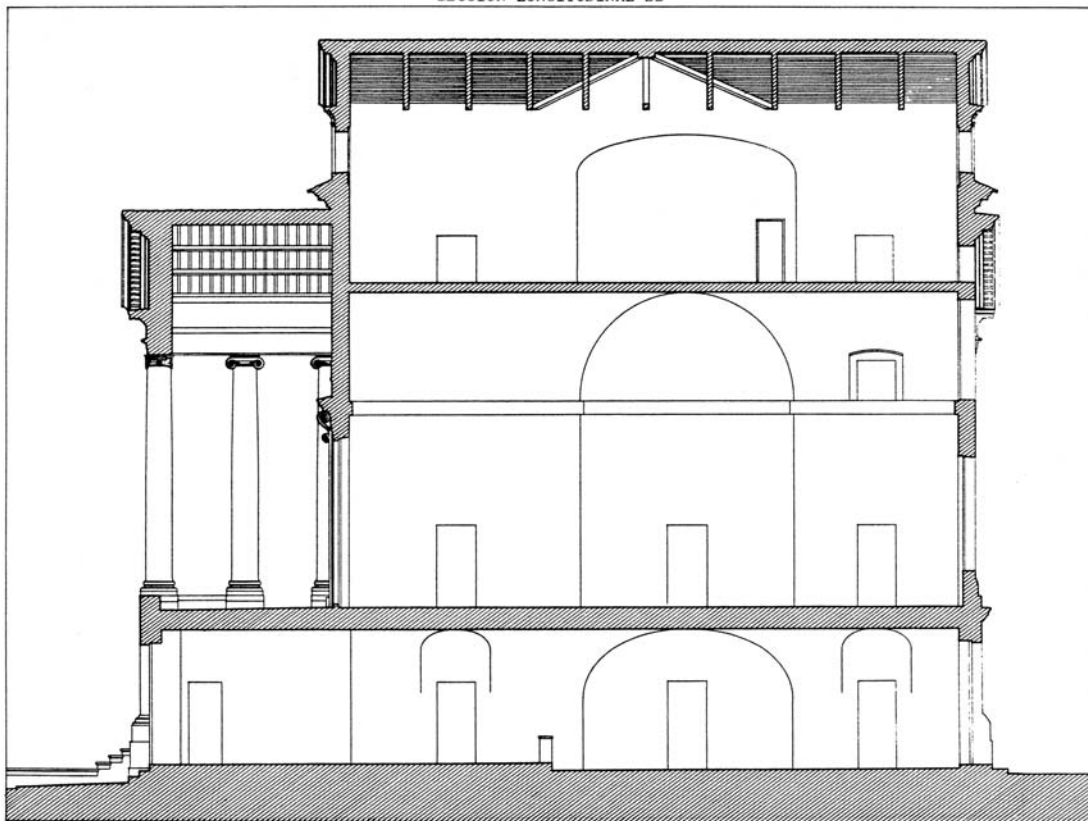
SECCION LONGITUDINAL BB
