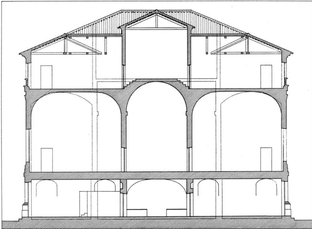
SECCION TRANSVERSAL AA
